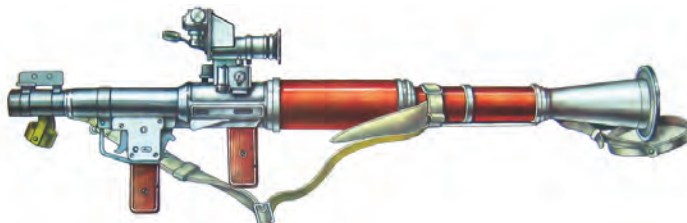
121-сурет. РПГ-7Д танкке қарсы қол гранатаметі.
