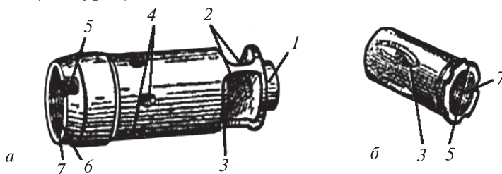
92-сурет. Ауыз тормозы — алау сөндіргіш (а) және компенсатор (б): 1—үш бөлігі; 2—саңылаулар; 3—жарма; 4—сөндіруші тесіктер; 5—біріктіру үшін кеспе; 6—айналасына бүгілген бөлігі; 7—ішкі бұранда.
