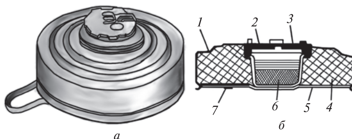
77-сурет. Танкке қарсы ТМ-62 М мина:
