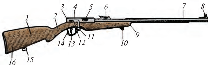
122-сурет. Шағын калибрлі мылтық (ТОЗ-8):
