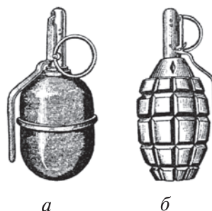
113-сурет. Бөлшектенуші қол гранаталарының жалпы көрінісі: а—РГД-5 гранатасы; б—Ф-1 гранатасы.
