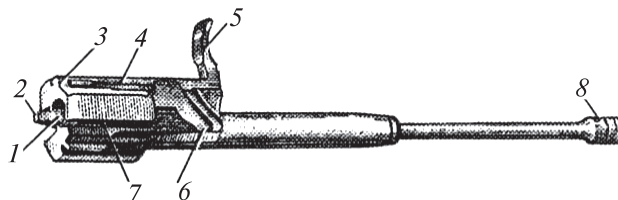
96-сурет. Затвордың рамасы, газ поршенімен бірге: 1—затвор үшін канал;
