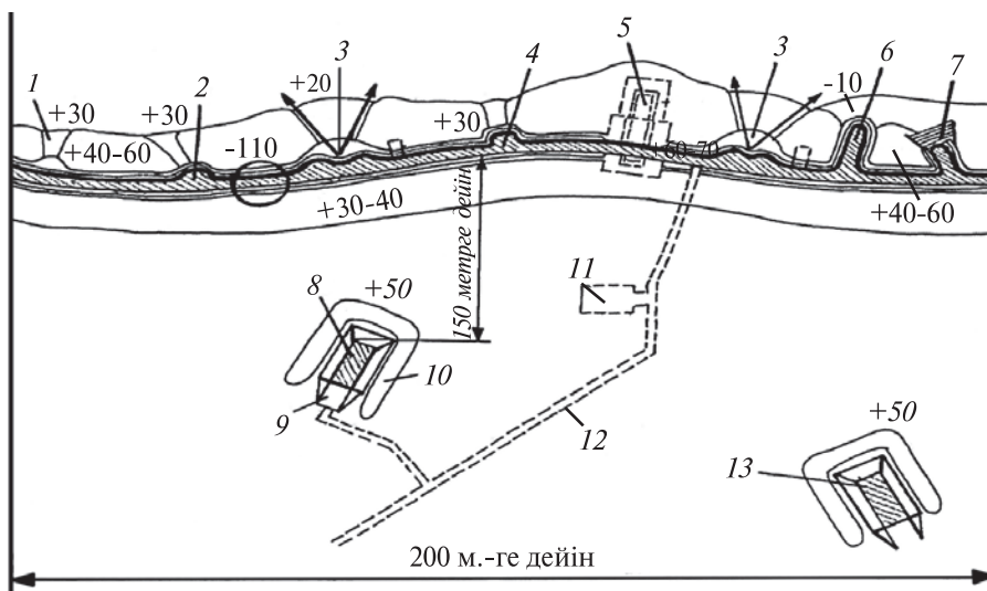
73-сурет. Окоптағы секция: 1—ұрыс алып бара жатқан ашықтық; 2—жан тараптарға өту; 3—пулеметтер үшін орын; 4—ату үшін орын; 5—үсті жабылған бекініс; 6—гранатамет үшін орын; 7—үсті жабылған ұрыс алып баратын ашықтық; 8—негізгі от ашу позициясында БМП үшін орын; 9—аппарель; 10—топырақ үйіндісі; 11—қажеттілік жайы; 12—байланыс жолдары; 13—запаста от ашу жағдайындағы БМП үшін орын.
