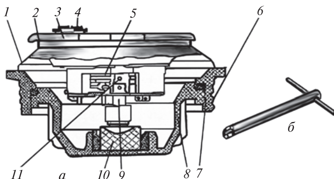
78-сурет. МВЧ-62 жарылғыш:
