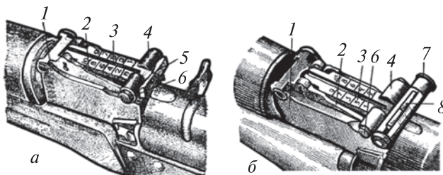
95-сурет. Нысанаға алу құрылғысы: а—автоматқа орнатылатын; б—пулеметке орнатылатын; 1—құрылғы негізі; 2—құрылғы жолақтары; 3—планка; 4—жүретін шығыршық; 5— нысана планкасының аяғы; 6—жүруші шығыршық тартқысы; 7—нысана винтінің бұрағышы; 8—нысана.
