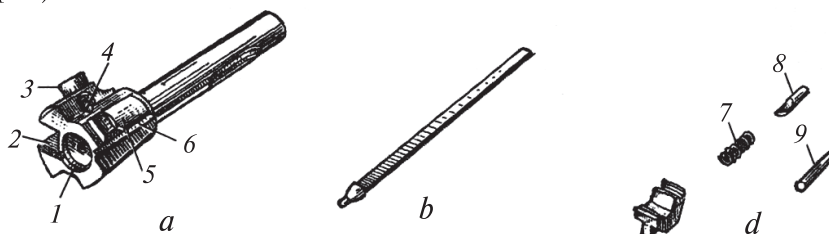
97-сурет. Затвор: а—затвордың негізі; б—соққы; д—лақтырғыш; 1—гильза үшін
