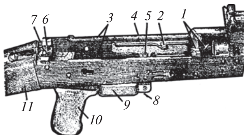
93-сурет. Ствол қорабы: 1—кеспелер; 2—қайтарушы дөнес; 3—бөртпелер; 4—бағыттаушы бөртпе; 5—біріктіруші; 6—балама аралық; 7—көлденең аралық; 8—магазин үшін арналған қыстырғыш; 9—тепкінің шығыршығы; 10—пистолет тұтқасы; 11—дүм.
