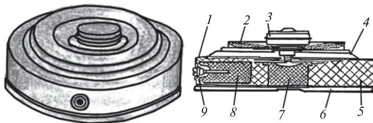
74-сурет. Танкке қарсы ТМ-57 мина МВЗ-57 жарылғышпен бірге көрінісі: а — транспорт түріндегі жалпы көрінісі, б — жауынгердің түріндегі минаның кеспеде көрінісі; 1—корпусы; 2—қалқан; 3—МВЗ-57 жарылғыш; 4—диафрагма (перделі тосқауыл); 5—заряды; 6—асты; 7—орталық детонатор; 8—жанындағы детонатор; 9—қақпағы.
