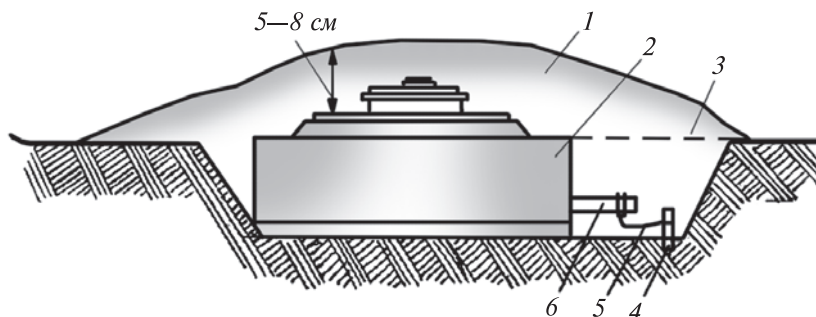
76-сурет. Танкке қарсы минаның жайдақ жерлерде орнатылуы: 1—бүркенуші қабат; 2—мина; 3—мина топырақ өлшемі; 4—қазық; 5—біріктіруші; 6—бүйір жарылғыш.
