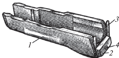
101-сурет. Стволдың астыңғы қаптамасы (тұтқасы): 1—бармақтар үшін жай; 2—бөртпе; 3—тегіс пружина; 4—шомпол үшін тесік.
