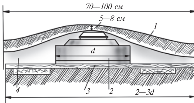
79-сурет. Танкке қарсы минаның жұмсақ (ылғалды) жерде орнатылуы:
