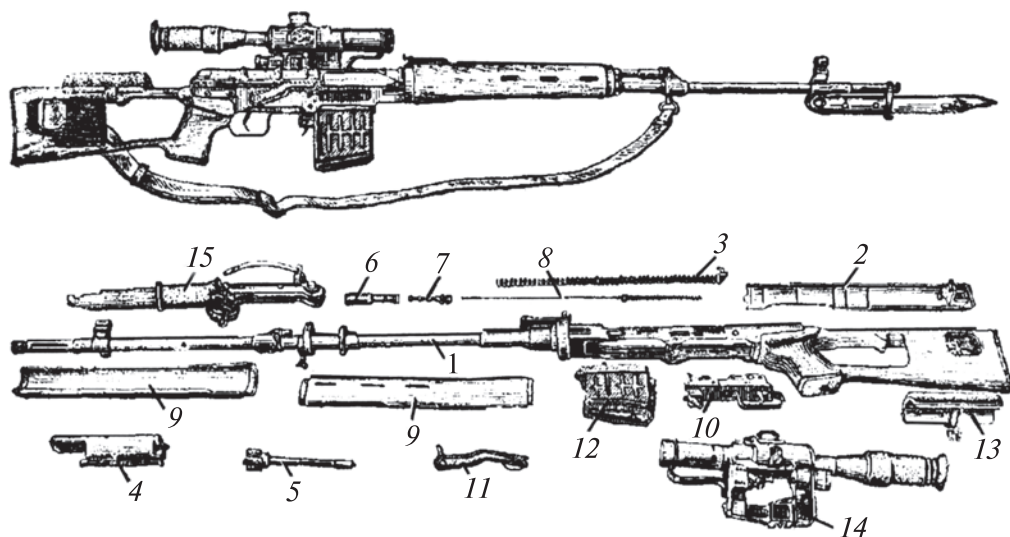
119-сурет. СДВ-нің жалпы көрінісі, негізгі бөлім және механизмдері:
