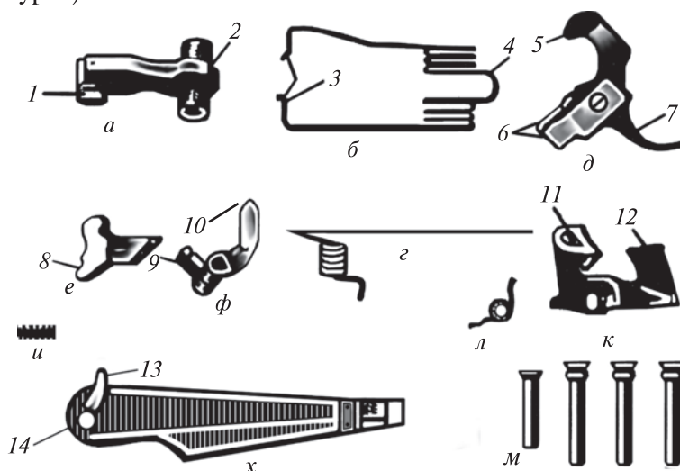
100-сурет. Соққылы тепкі механизмінің бөлшектері: а—тепкі; б—жауынгерлік пружина; д—ілмек; е—жеке түрде от ашу шепталосы; ф—автотепкі; г—автотепкі пружинасы; х—өткізгіш; и—жеке тәрізде от ашу шепталосының оқтары мен пружиналары; к—тепкі әрекетін сөндіруші; л—тепкінің әрекеті сөндіргішінің пружинасы; м—құбыр сияқты ок. 1—жауынгерлік беті; 2—автотепкі беті; 3—бүгілген ұштар; 4—топса; 5—кисық бөртпе; 6—тура бұрышты бөртпелер; 7—дүмше; 8—кеспе; 9—шаптало; 10—тіргек; 11—зашелка; 12—алдыңғы бөртпе; 13—өткізуші бөлігі; 14—сапфа.
