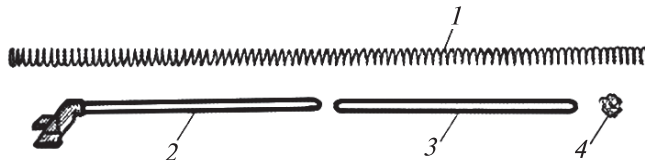
98-сурет. Қайтарушы механизм: 1—қайтарушы механизм; 2—бағыттаушы таяқша; 3—әрекеттенуші таяқша; 4—муфта (окты жолдаушы).
