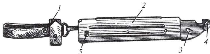
104-сурет. Кын: 1—ілгіш, сырмалы белдік және карабинмен бірге; 2—пластмассалы қабық; 3—оқ бөртпе; 4—тірек; 5—тегіс пружина біріктіргіші.
