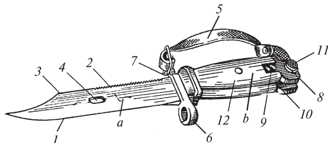
103-сурет. Найза-пышақ: a —жүз; b —тұтқа; 1—кесетін кыры; 2—ара; 3—өткірленген жүзі; 4—тесік; 5—белдік, 6—шығыршық; 7—белдік үшін ілгіш; 8—тұтқаның металл бөлігі; 9—қосатын винт; 10—бойлама кеспе; 11—тартқы; 12—сап.
