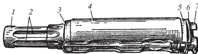
99-сурет. Газ трубкасы ствол қаптамасымен бірге: 1—газ трубкасы; 2—газ поршені үшін бағыттаушы қабырғалар; 3—алдындағы біріктіргіш; 4—стволдың үстіңгі қаптамасы; 5—артқы біріктіруші; 6—бөртпе, 7—тегіс пружина.
