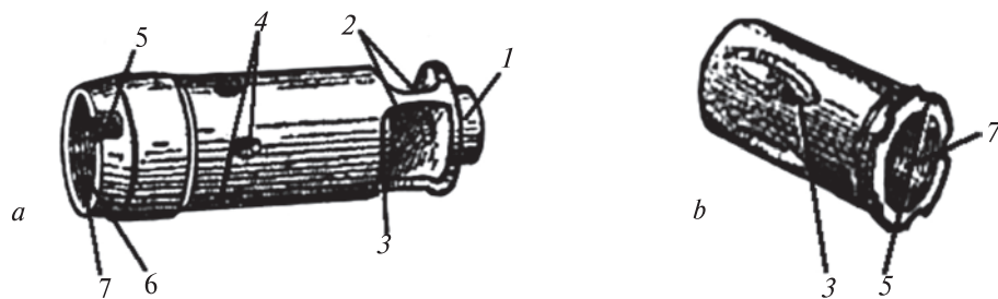
92-súwret. Awız tormozı — jalın sóndirgish (a) hám kompensator (b):
