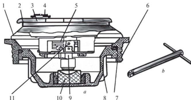
78- súwret. MVCH-62 jarǵıshı.
