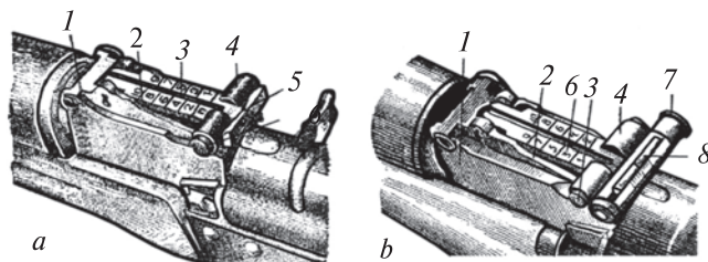
95-súwret. Nishangá alıw úskenesi:
