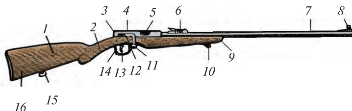
122- súwret . Kishi kalibrli miltıq (TOZ-8):
