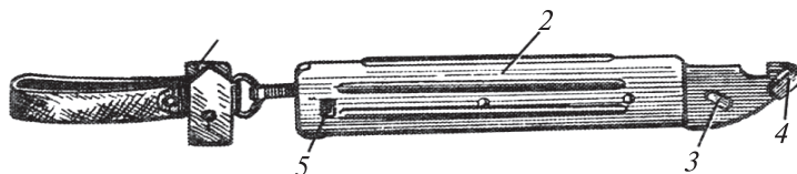
104-súwret. Qın: 1 — ildirǵış, ilmekli remen hám karabin menen birgelikte; 2 — plassmassalı qabı; 3 — oq-bórtpe; 4 — tayanshı; 5 — jalpaq prujına biriktiriwshi.
