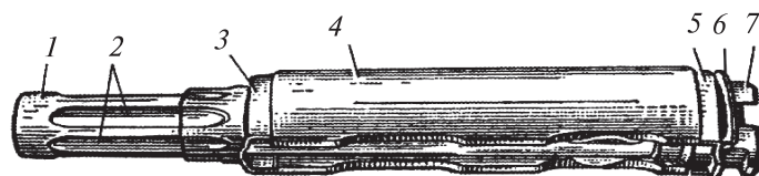
99-súwret. Gaz trubkası stvol qaplaması menen birge: 1—gaz trubkası; 2—gaz porsheni ushın baǵdarlawshı qabırǵalar; 3—aldıńǵı biriktiriwshi; 4—stvol ústi qaplaması; 5—artqı biriktirgish; 6—bórtpe; 7—jalpaq prujina.
