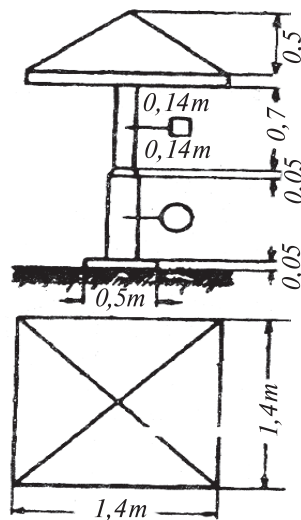
Saqshı minarasi jayınıń rejesi.
