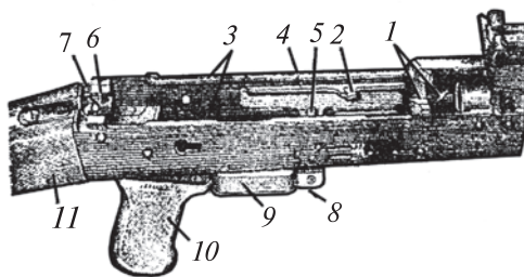
93-súwret. Stvol qutısı: 1 — kespeler; 2 — ılaqtırıwshı bórtpе; 3 — dúńki; 4 — baǵdarlawshı bórtpе; 5 — biriktirgish; 6 — biyiklik aralıq; 7 — kese aralıq; 8 — magazin qıstırǵıshı; 9 — tepki shúrppesi; 10 — pistolet tutqası; 11 — qundaq.
