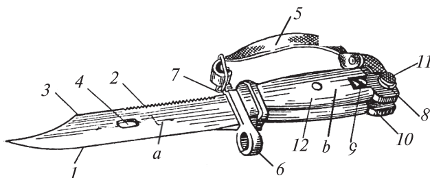
103-súwret. Nayza-pışhaq : a — tıyǵı; b — tutqası; 1 — kesiwshi júzi; 2 — jargı; 3 — sharxlangan ushı; 4 — tesik; 5 — remen; 6 — saqıyna, 7 — remen ushın ilǵış, 8 — dásteniń metall bólimi, 9 — biriktiriwshi vint, 10 — uzınsha kespe, 11 — tartqı, 12 — dáste.
