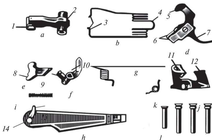
100-súwret. Soqqı beriwshi-tepki mexanizminiń bólekleri.
