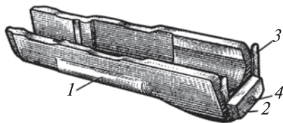
101-súwret. Stvol astı tutqası (cevyo): 1 — barmaqlar ushın orın; 2 — börtpe; 3 — jalpaq prujına; 4 — shompol ushın tesik.
