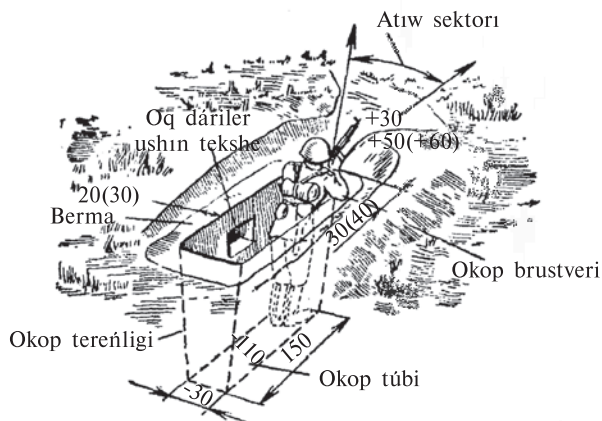
51-súwret. Avtomattan dizerlep otırıp atıw ushın okop.
