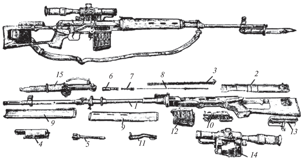
119-súwret. SDVnıń ulıwma kórinisi, tiykargı bólim hám mexanizmleri:
