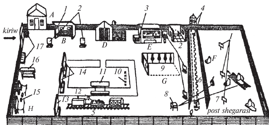
7-súwret. Jeke quramdı xızmetti ótewge tayarlaw ushın qarawıl qalashasın úskenelew:
