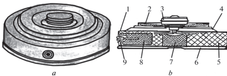
74-súwret. Tankke qarsı TM-57 minası MVZ-57 jarıwshı menen birge kórinisi:
