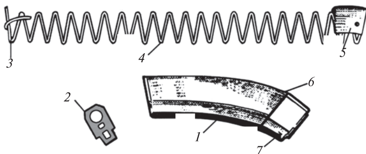
102-súwret. Magazin: 1 — korpus; 2 — qaqpaq; 3 — bekkemlewshi planka; 4 — prujına; 5 — jiberiwshi; 6 — tayanısh börtpesi; 7 — ilgish.
