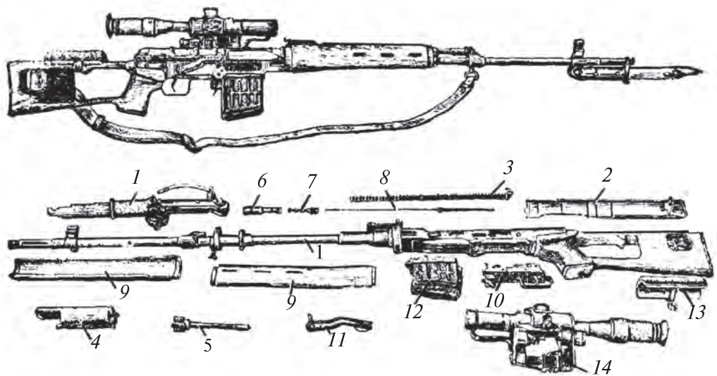
119-njy surat. SDV-nyň umumy görnüşi, esasy bölekleri we mehanizmleri: 1—stwol gutusy aýyk nyşana alyjy gundagy bilen bilelikde; 2—stwol gutusynyň gapagy; 3—gaýtaryjy mehanizm; 4—zatwor ramasy; 5—zatwor; 6—gaz trubkasy regulýatory bilen; 7—gaz porşeni; 8—iteriji puržin bilen; 9—stwol örtükleri; 10—naýça depgi mehanizmi; 11—saklaýjy; 12—magazin; 13—gundagyň üsti; 14—optiki nyşana alyjy; 15—naýza-pyçak.
