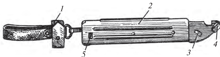
104-nji surat. Gyn: 1—ilgençek, halkaly kemer we karabin bilen bilelikde; 2—plastmassaly daşlyk; 3—ok-çykyt; 4—daýanç; 5—ýasy puržin birikdiriji.
