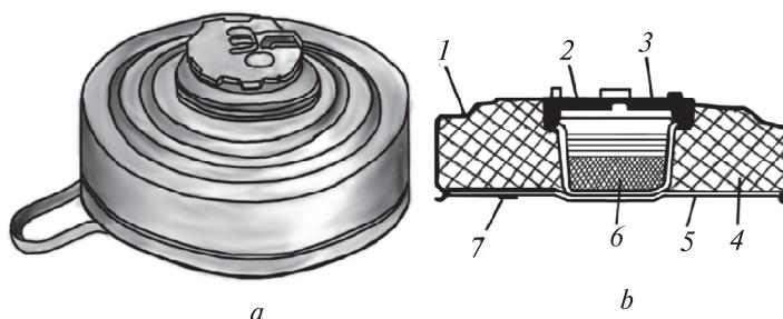
77-nji surat. Tanka garşy TM-62 M mina:
