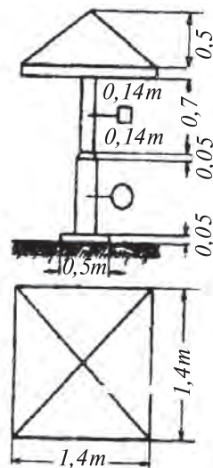
Sakçy minarasynyň üçeginiň plany.
