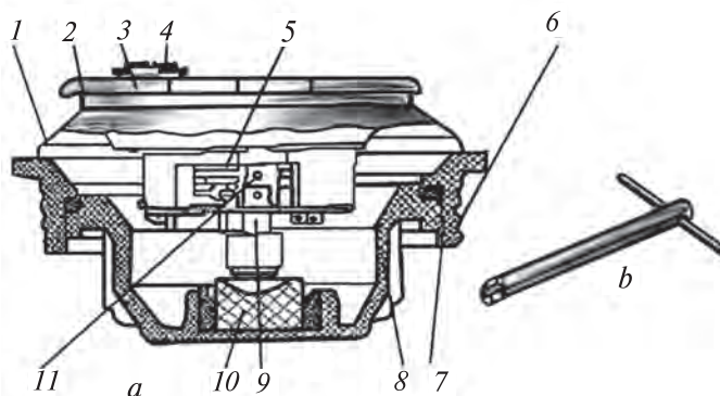
78-nji surat. MVCH-62 partladyjy:
