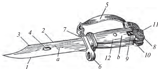
103-nji surat. Naýza-pyçak: a —tyg; b —dasta; 1—kesiji gyraň; 2—byçgy; 3—ýteldilen ujy; 4—deşik; 5—kemer; 6—halka; 7—kemer üçin ilgençek; 8—dessäniň metal bölegi; 9—goşujy wint; 10—dik kesik; 11—çeki; 12—sop.
