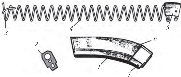
1—korpus; 2—gapak; 3—berkidiji planka; 4—puržin; 5—goýberiji; 6—daýanç cykydy; 7—ilgençek.
