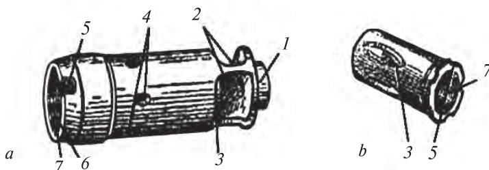
92-nji surat. Agyz tormozy — ot söndüriji (a) we kompensator (b): 1—uçky bölegi; 2—deşikleri; 3—ýaryk; 4—söndüriji yşlar; 5—birikdiriji üçin kesik; 6—töwerekleýin eplenen bölegi; 7—içki hyr.
