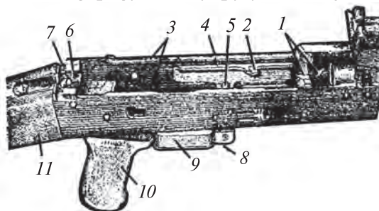
93-nji surat. Stwol gutusy: 1—kesimler; 2—gaýtaryjy çykyt; 3—çykytlar; 4—ugrukdyryjy çykyt; 5—birikdiriji; 6—dik aralyk; 7—kese aralyk; 8—magazin üçin nyşana alnan ildirgiç; 9—depgi halkasy; 10—pistolet dessesi; 11—gundak.
