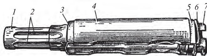
99-njy surat. Gaz trubkasy stwol örtügi bilen bilelikde: 1—gaz trubkasy; 2—gaz porşeni üçin ugrukdyryjy gapyrgalar; 3—öňdäki birikdiriji; 4—stwol üsti örtügi; 5—yzky birikdiriji; 6—çykyt; 7—ýasy puržin.
