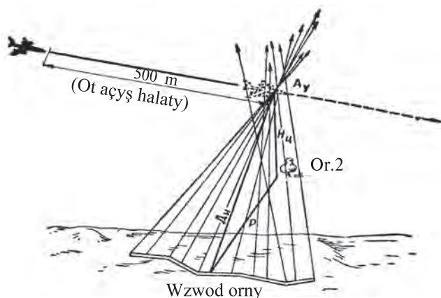
Wzvod orny 52-nji surat. Samolýotlara böwetli ot açyş.
