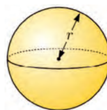
Шар
