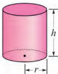
Цилиндр
