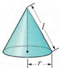
Конус
