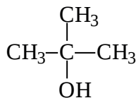
2-метилпропанол-2 үчүнчүлүк спирт
