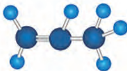
Пропен ( C_3H_6 )
