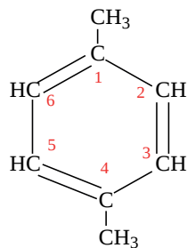
1,4-диметилбензол (p-ксилол)
