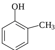
фенол
