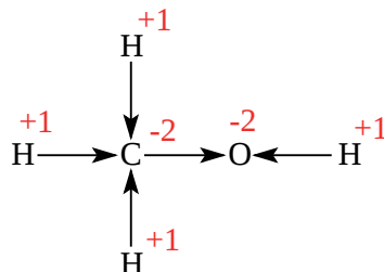
метанол
