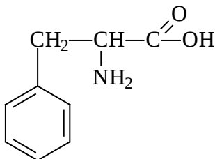
фенилаланин
