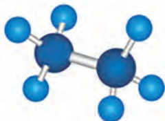
этан
