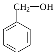
бензил спирти
