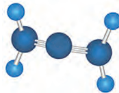
Пропadiен ( C_3H_4 )
