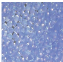
Полиэтилен
