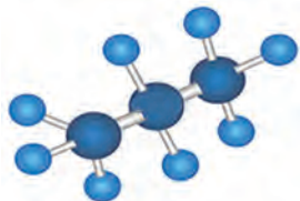
Пропан ( C_3H_8 )
