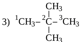
2,2-диметилпропан
