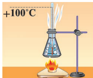
16-njy surat. Suw +100^{\circ}\text{C} -da gaýnaýar.
