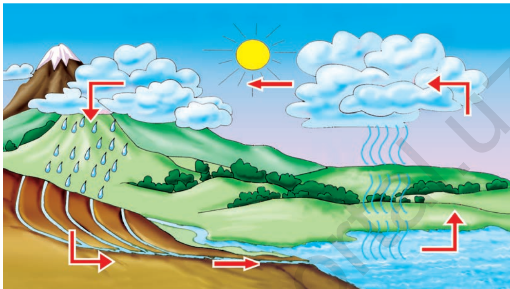
23-nji surat. Tebigatda suwuň aýlanyşy.
