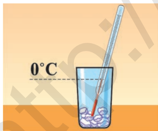
14-nji surat. Buz 0^{\circ}\text{C} -da ereýär.
