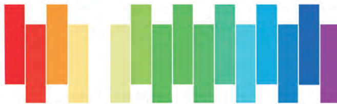
Ren'li spektr
