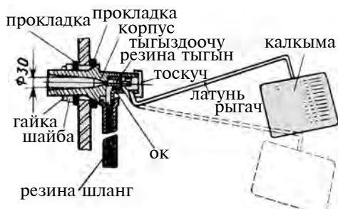
82-сүрөт. Калкыма клапандын түзүлүшү.
