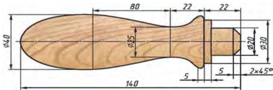
32-сурет. Өгөө туткасынын өлчөмдөрү.
