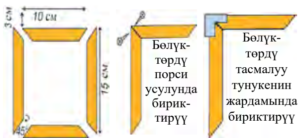
21-сүрөт. Рамканын чиймеси.
