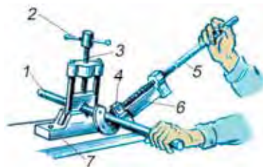
62-сүрөт. Түтүк кескичте иштөө: 1 – түтүк; 2, 5 – туткалар; 3 – винт; 4 – кыймылдуу ролик; 6 – кескич; 7 – кыскыч.
