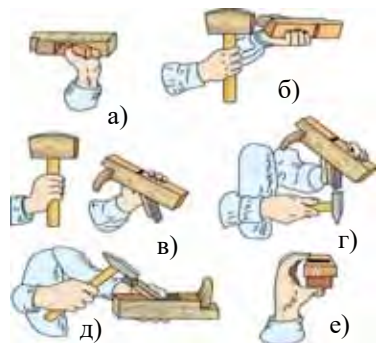
8-сүрөт. Сүргүнү ишке даярдоодо бычакты корпустан чыгаруу жана кайра орнотуу: а, б – бычакты чыгарууда корпус ушундай кармалат; в, г – бычакты корпуска орнотуу; д – шынааны бекемдөө; е – бычактын туура орнотулгандыгын текшерүү.
