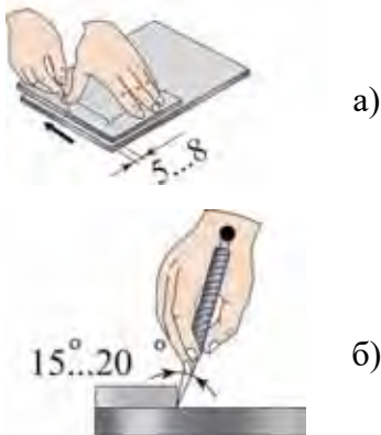
46-сүрөт. Чийме боюнча тик бурчтуу деталдарды пландоо.
