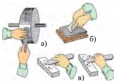
9-сүрөт. Сүргүнү ишке даярдоодо бычакты курчутуу жана кайроо; а – курчутуу; б – кайроо; в – кылоолоо.
