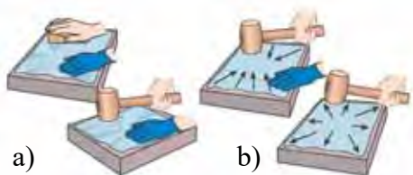
45-сурет. Түніке листерін тегістеу ережелері.
