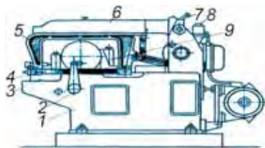
61-сурет. Аралау станогы: 1 – станина; 2 – тіреуіш; 3 – орындық; 4 – ара полотносы; 5 – аралау рамасы; 6 – сық (оқ); 7 – айырып-қосқыш; 8 – кнопка (іске қосу-тоқта); 9 – машина қысқышы.
