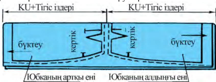
44-сурет. Тура пішімді юбканың өлшемін матаға жайғастыру.
