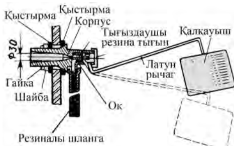
82-сурет. Қалтқылы кранның түзілісі.
