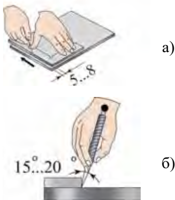
46-сурет. Сызба бойынша тік бұрышты деталдарды жоспарлау
