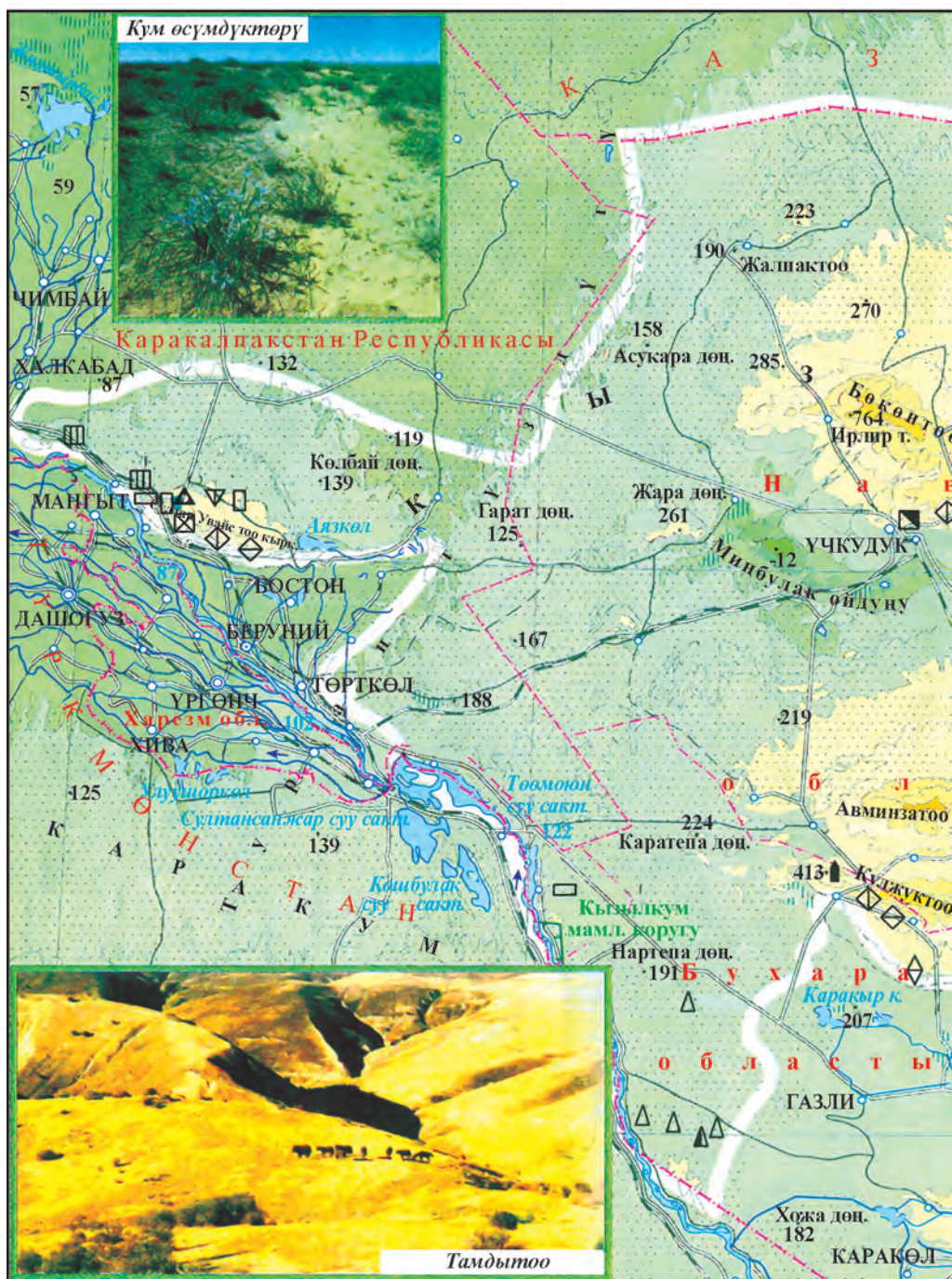
42-сүрөт. Кызылкум табигый
