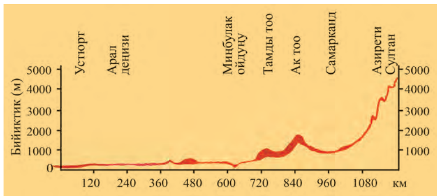
28-сүрөт. Миңбулак ойдуңу менен Азирети Султан чокусу аркылуу өткөн жер бетинин жара кесилиши.
