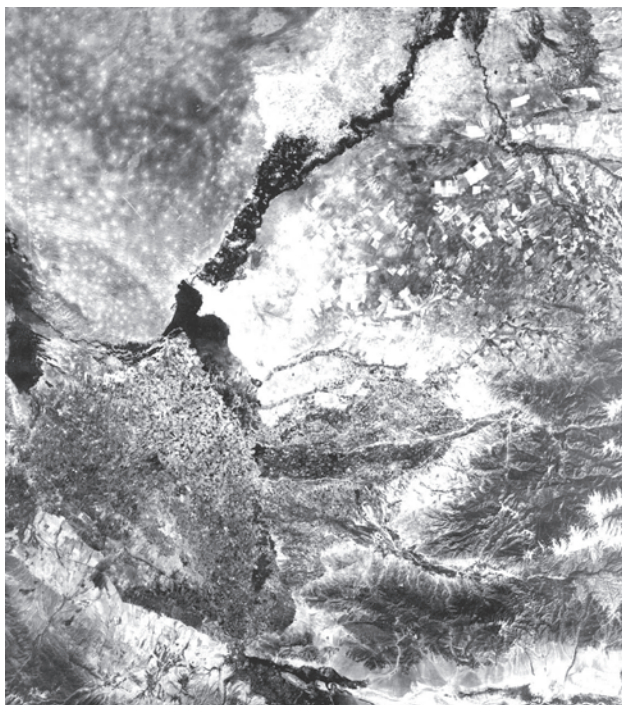
5-сүрөт. Мырзачөл жана Ташкент оазисинин космосүрөтү.
