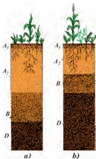
19-сүрөт. Топурак кесиндилери:
