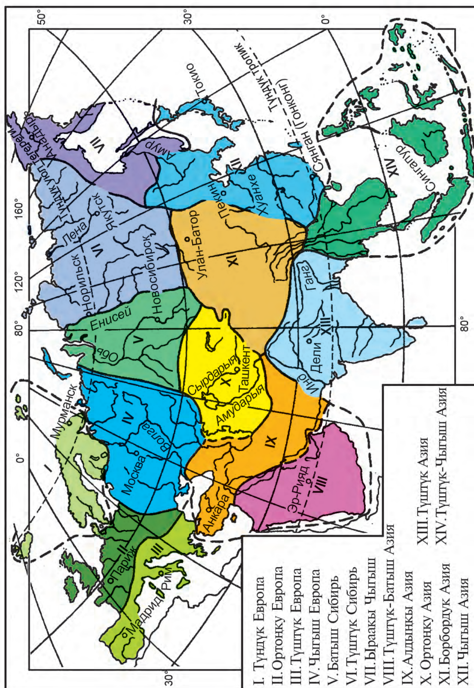
1-сүрөт. Евразиянын табигый географиялык чөлкөмдөрү.
