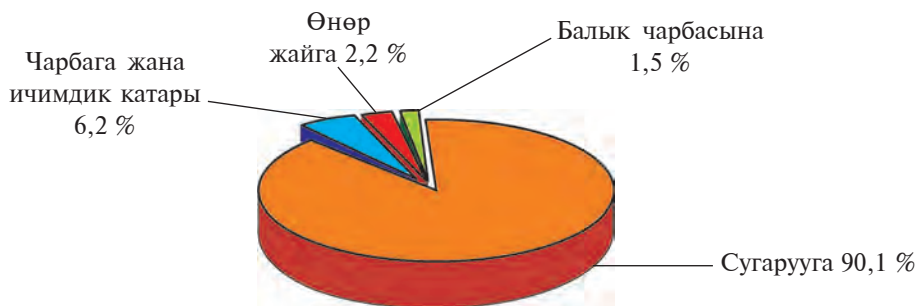
31-сүрөт. Ўзбекстанда пайдаланыла турган суулардын бөлүштүрүлүшү.
