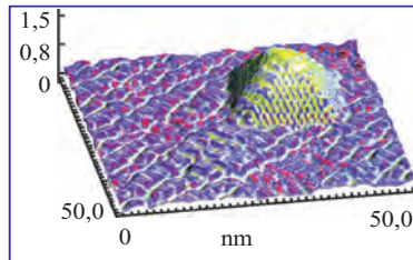
8-сурет. Германий атомының кремний құрылысының арасында орналасуы.
