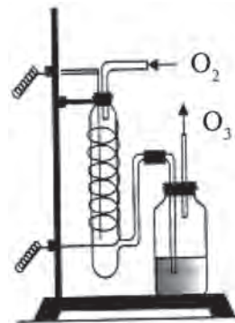
21-сурет. Озонатор
