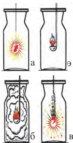
22-сурет. Оттегінің химиялық қасиеттері Көмірдің (а), күкірттің (ә), фосфордың (б) және темірдің (в) оттегіде жануы.
