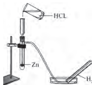
28-сурет. \text{Zn} -тың \text{HCl} -нан сутегіні ығыстырып шығаруы.
