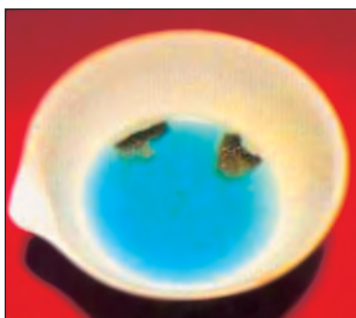
46-сурет. Мыс және басқа кейбір металдардың түрлі қышқылдармен әсерлесуі.
