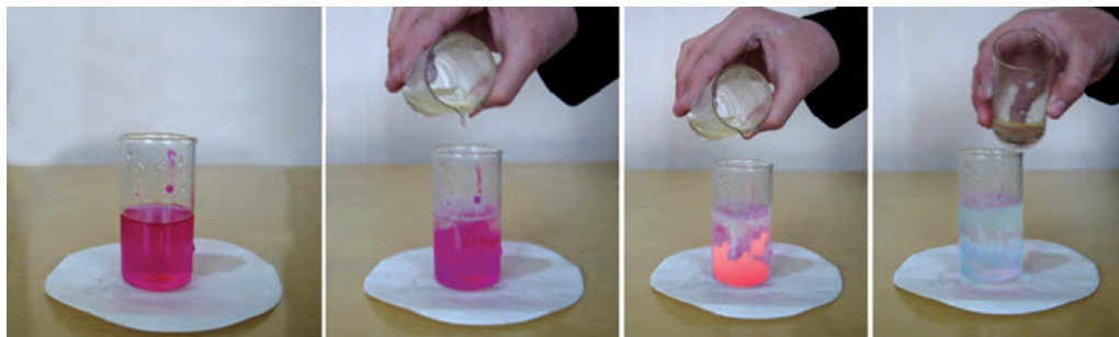
44-сурет. Фенолфталеинді сілті ерітіндісін қышқыл ерітіндісімен нейтралдауда индикатор түсінің жойылуы.
