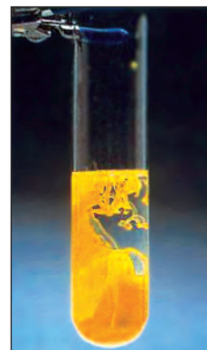
Рис.52. Образование осадка \text{AgI} при взаимодействии \text{AgNO}_3 с \text{NaI}
