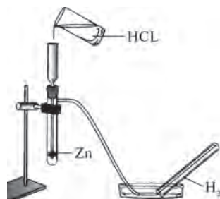
Рис.28. Вытеснение водорода цинком из соляной кислоты
