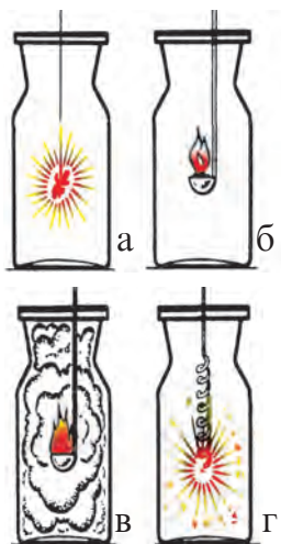
Рис.22. Химические свойства кислорода: горение в кислороде угля (а), серы (б), фосфора (в), железа (г).
