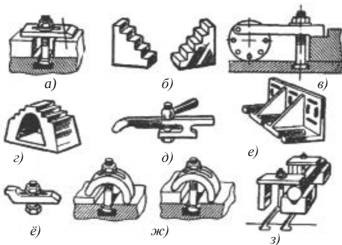
37-сүрөт. Фрезерлөө станогунда заготоканы орнотуунун удаалаштыгы.
