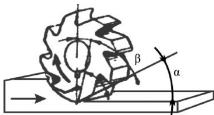
35-сүрөт. Фрезанын негизги бурчтары.
