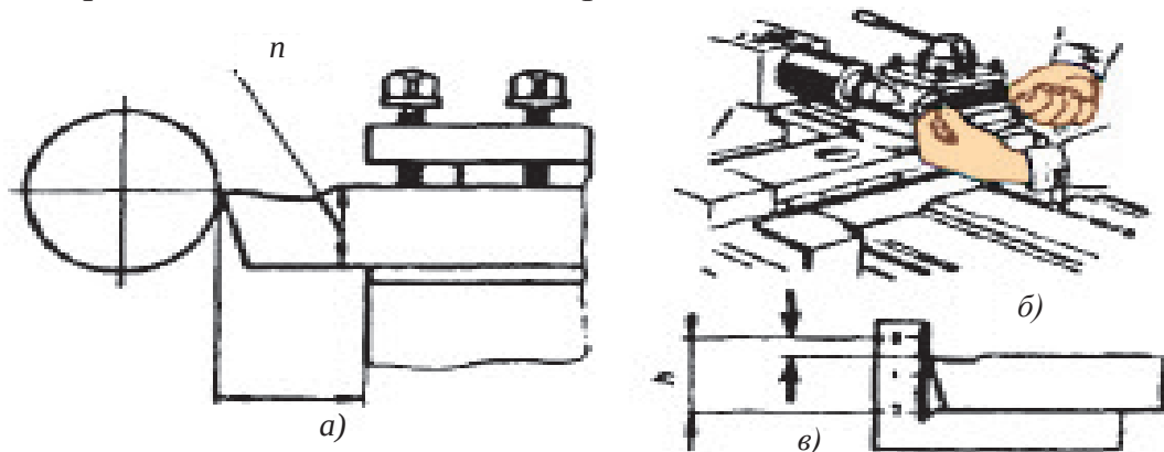
45-сүрөт. а – кескич жана кескичти кармагыч; б – кескичтин бийиктигин текшерүү; в – бурчтуу шаблон.
