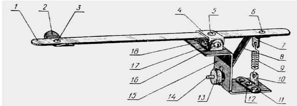
59-сүрөт. Реленин туташтыруучу механизми: 1 – якорь; 2 – контакт пластинасы; 3 – бөрк; 4 – якорь илмеги; 5, 6 – бөрк; 7 – үстүңкү кронштейн; 8 – чектегич; 9 – пружина; 10 – астыңкы кронштейн; 11 – бөрк; 12 – винт; 13 – гайка; 14 – винт; 15 – Z сымал стойка; 16 – винт; 17 – стойканын илмеги.
