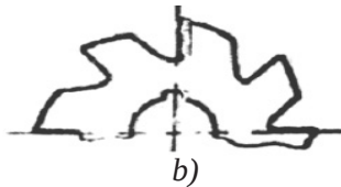
34-сурет. Фрезерлеу формасы: а – өткір шарықталған тісті; б – әшекейлейтін тіс.
