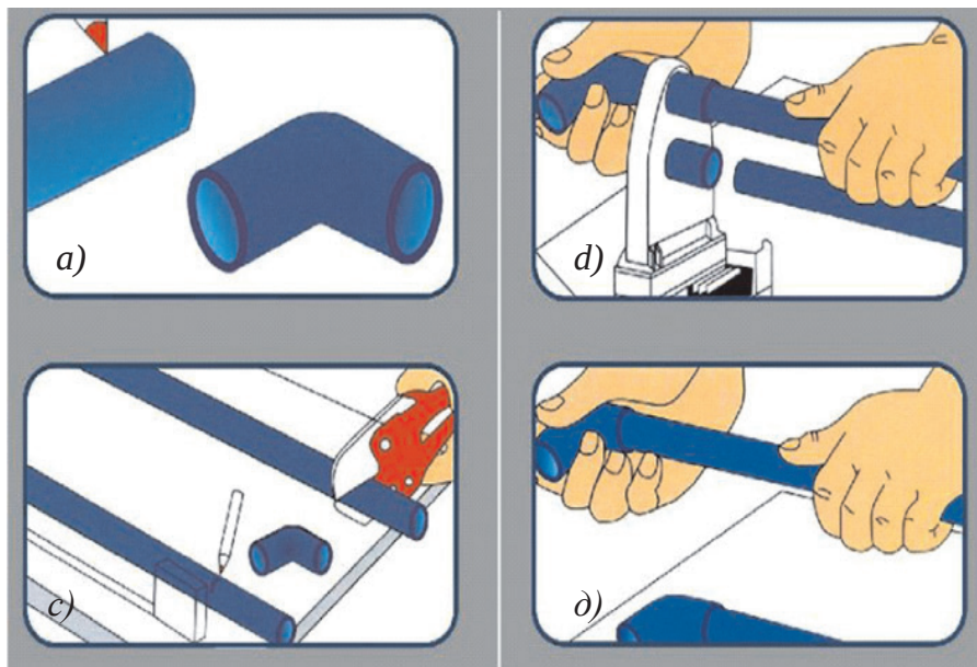
22-сурет. Пластмасса құбырды жалғау процесі.
