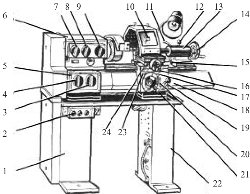
40-сурет. TV-6 винт ашатын токарлық станогы:
