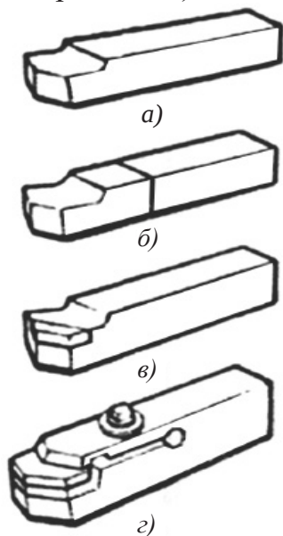
41-сурет. Кескіштер:
