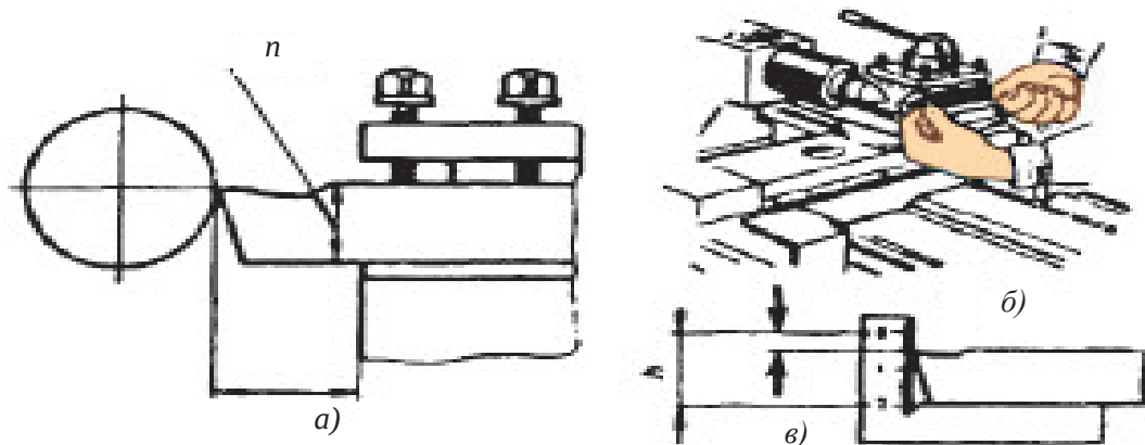
45-сурет. Кескіш ұстағышта; б) кескіштің биіктігін тексеру; в) бұрышты қалып
