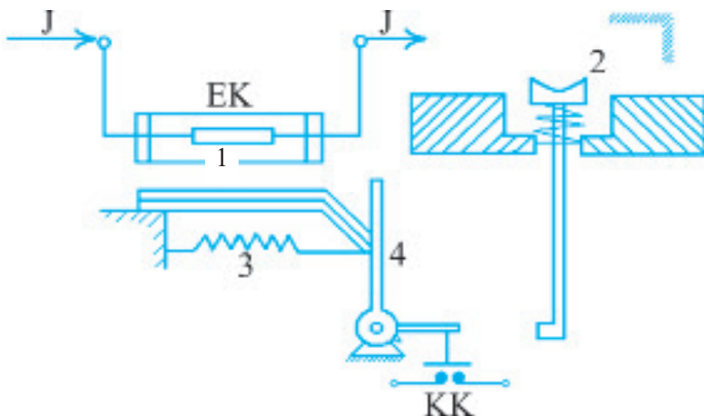
52-сурет. Жылулық релесінің түзілісі: 1 – биметалл жапырақ; 2 – қайта іске үсіруші түйме; 3 – пружина; 4 – биметалл жапырақ тұтқасы.
