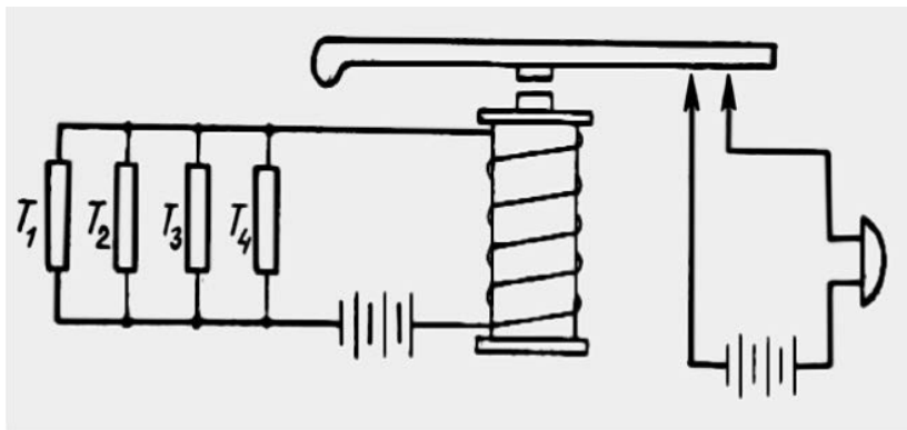
57-сурет. Өрттен хабар беруші автоматикалық сигнализация құрылмасы.
