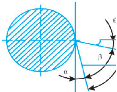
43-сурет. Кескіштің негізгі бұрыштары.
