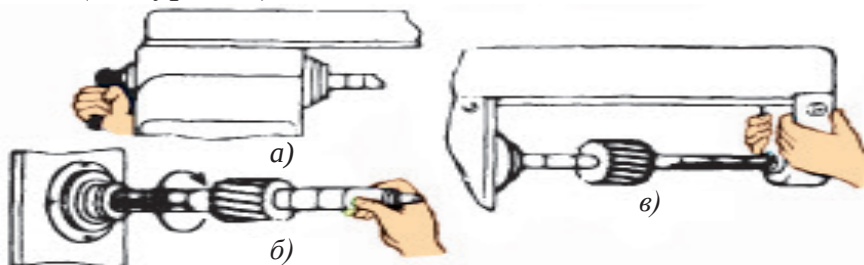
39-сурет. Цилиндрлі фрезаларды орнату; а) оправканы орналастыру; б) орнатушы шиырқыштарды орналастыру; д) шиыршықты орнату.
