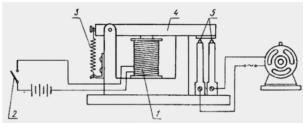
56-сурет. Электродвигателдің жұмысын басқару схемасы.
