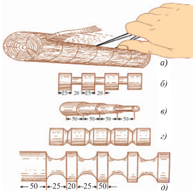
17-сурет. Әр түрлі беттерді жоспарлау және жону: а – циркуль көмегімен жоспарлау; б – тік бойындар жасау; в – баспалдақты беттер; г – ойлы кескіндер; д – майысқақ беттер.
