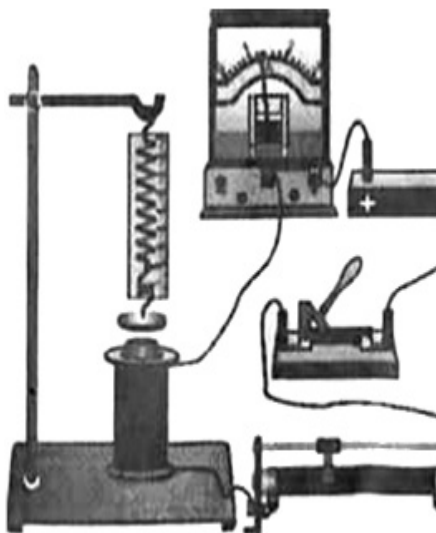
55-сурет. Электромагнит алаңының әсер күшін анықтау.
