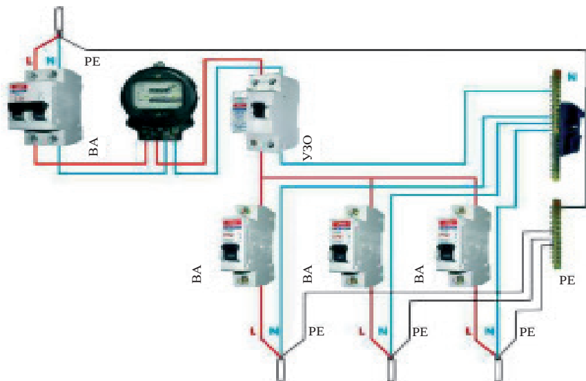
62-сурет. Үй электр қамтудың үлгілі схемасы.
