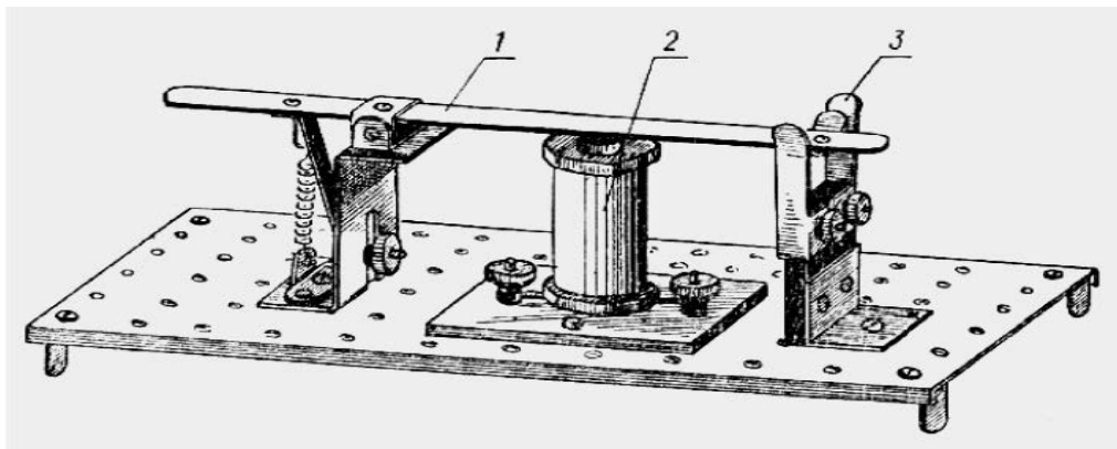
58-сурет. Электромагнитті реленің негізгі элементтері.
