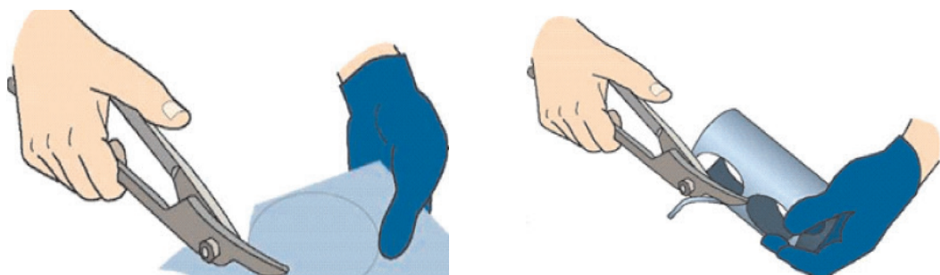
48-сурет. Қол қайшы мен жұқа лист материалды қырку.
