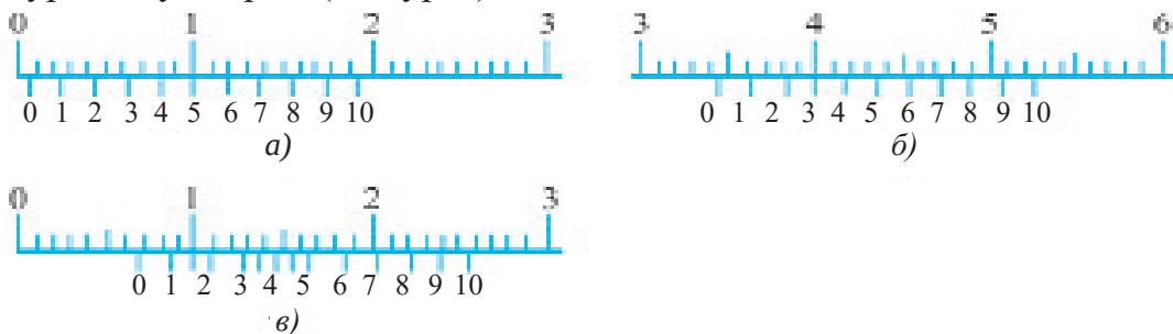
32-сурет. Штангенцикуль шкалаларының өлшеудегі жағдайы:
