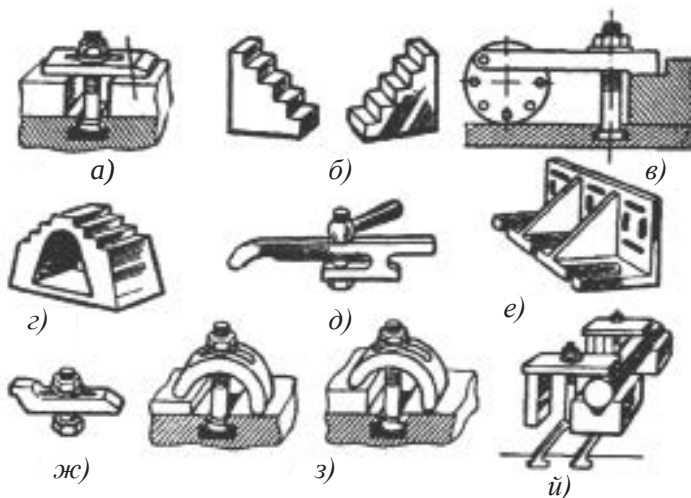
37-сурет. Фрезерлеу станогында дайындаманы орнату басқышы.
