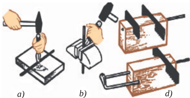
27-сурет. Сымды кескіш (а, б) және темір ара көмегімен қырқу (д)
