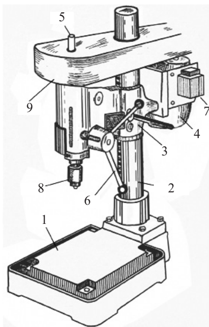
10-сурет. Бұрғылау станогы:
