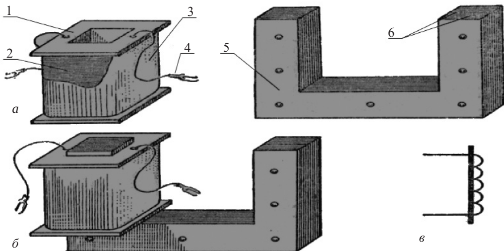
54-сурет. Электромагнит.
