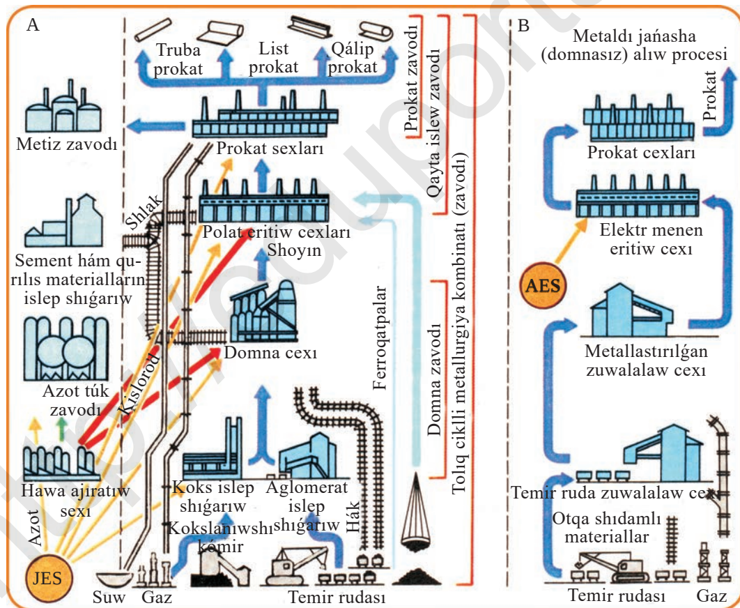
35-súwret. Metallurģiya kombinatındaǵı cexlar sxeması.
