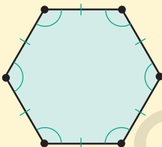
правильный шестиугольник
