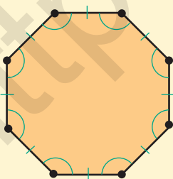
правильный восьмиугольник
