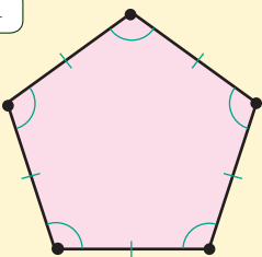
правильный пятиугольник
