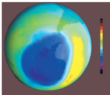
5-сүрөт. Антарктиданын үстүндө озон катмары жукарышынын схемалык көрүнүшү.
