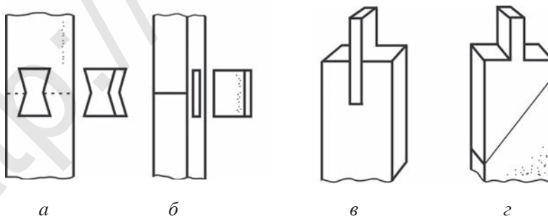
13-сурет. Мебель бөліктерін жөндеу: a – қаптама көмегінде ұзайттыру; б – тоғынды жөндеу; в, г – порси тәсілінде жөндеу.
