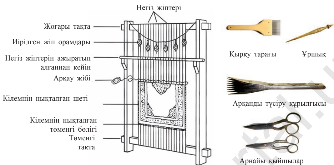
37-сурет. Кілем тоқу станогы және жұмыс құралдары.
