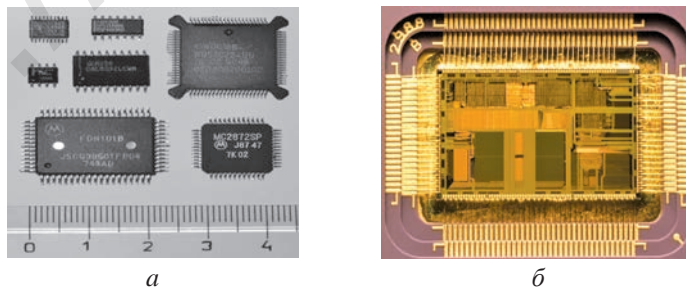
23-сурет. Цифрлы есептеу қондырғылары: a – интеграл микросхема корпусы; б – микропроцессор корпусы.
