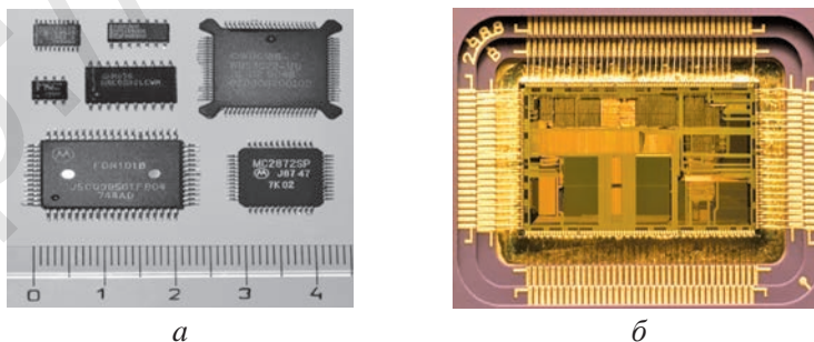
Рис. 23. Цифровые вычислительные установки: а – корпус интегральной микросхемы; б – корпус микропроцессора
