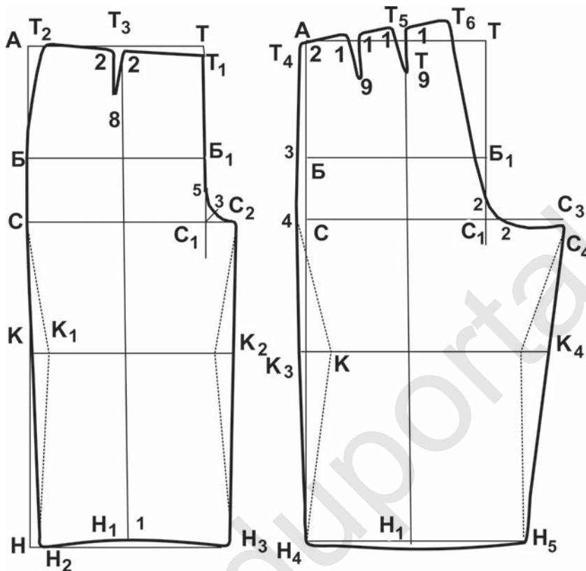
Рис. 41. Чертеж основы женских брюк
