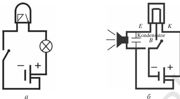
Рис. 22. Монтажная схема электрического звонка: а – для установки по передаче сигнала; б – для установки по приему сигнала
