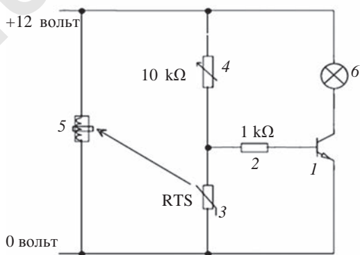
Рис. 19. Чертеж транзисторного ключа, к базе которого подключено термосопротивление: 1 – транзистор; 2 – резистор; 3 – терморезистор; 4 – резистор с преобразователем; 5 – нагреватель; 6 – лампочка
