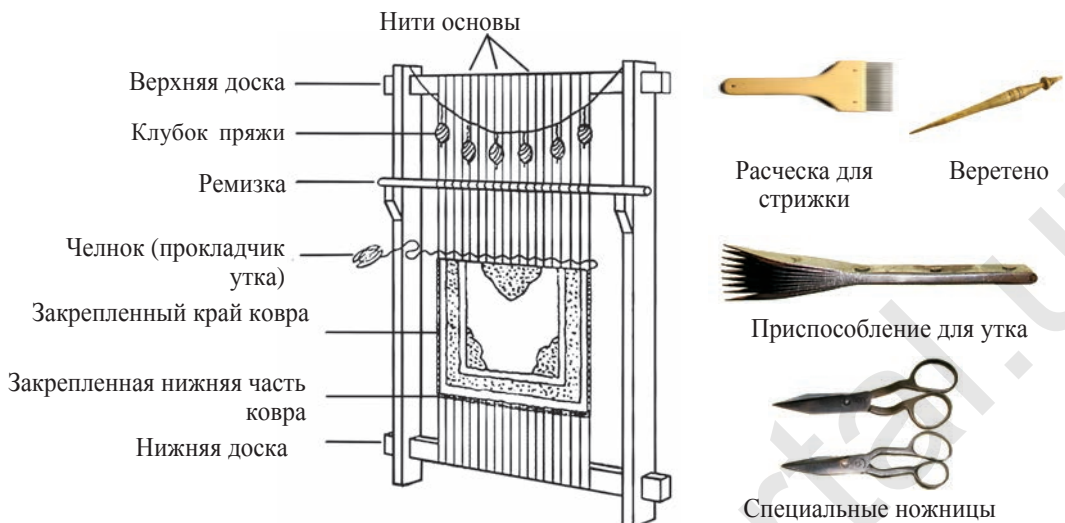
Рис. 37. Ковроткацкий станок и рабочие инструменты
