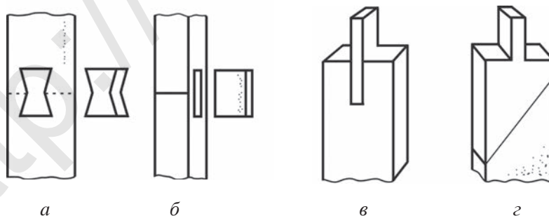
Рис. 13. Ремонт частей мебели: а – удлинение с помощью покрытия; б – ремонт скобы; в , г – ремонт методом частичной замены
