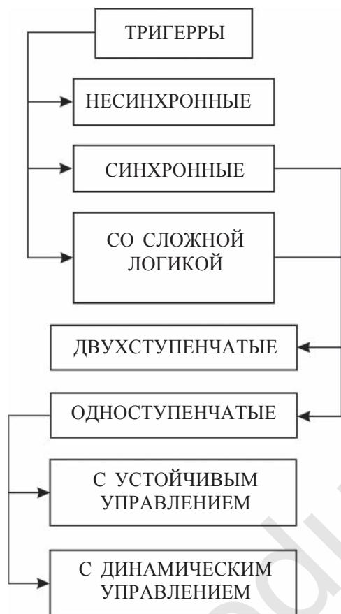
Рис. 24. Классификация триггеров по способу ввода данных
