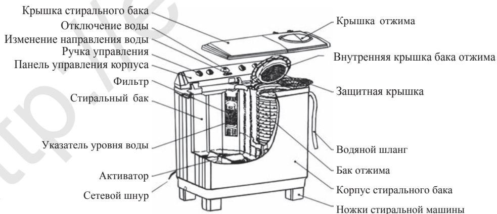
Рис.14. Строение полуавтоматической стиральной машины
